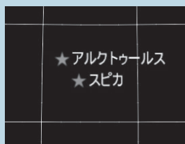
5万年後の夫婦星イメージ (ステラナビゲータ)
