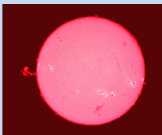
(望遠鏡で見た太陽表面：右側に黒点)
