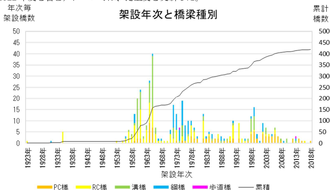
図-1.2.1 架設年次別施設の現状
