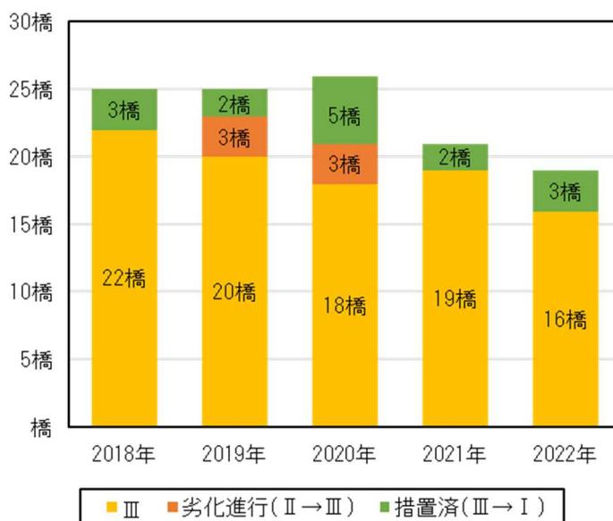
図-1.2.6 年度別Ⅲ判定橋梁の推移
