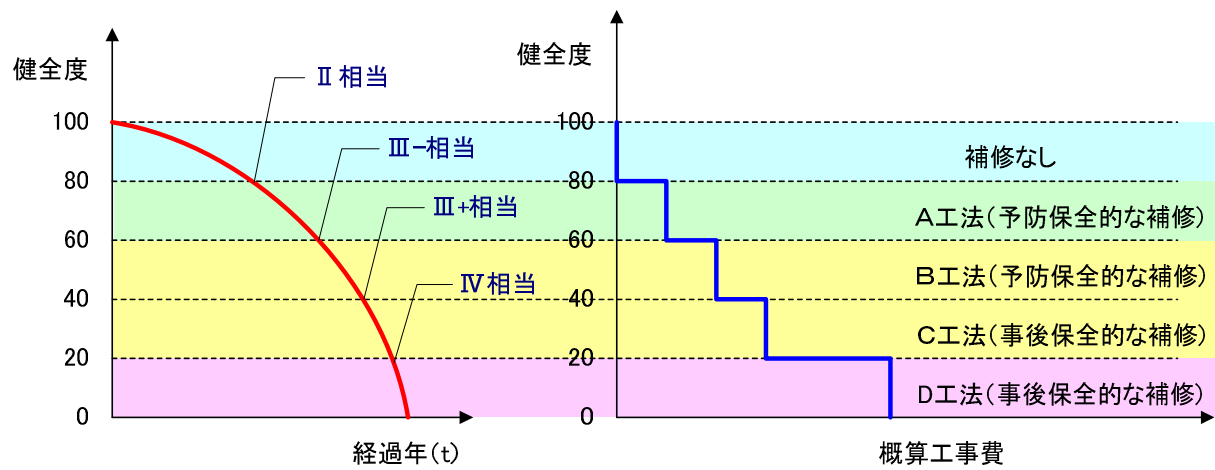
図-2.4.3 健全度と対策工法の概算工事費のイメージ
