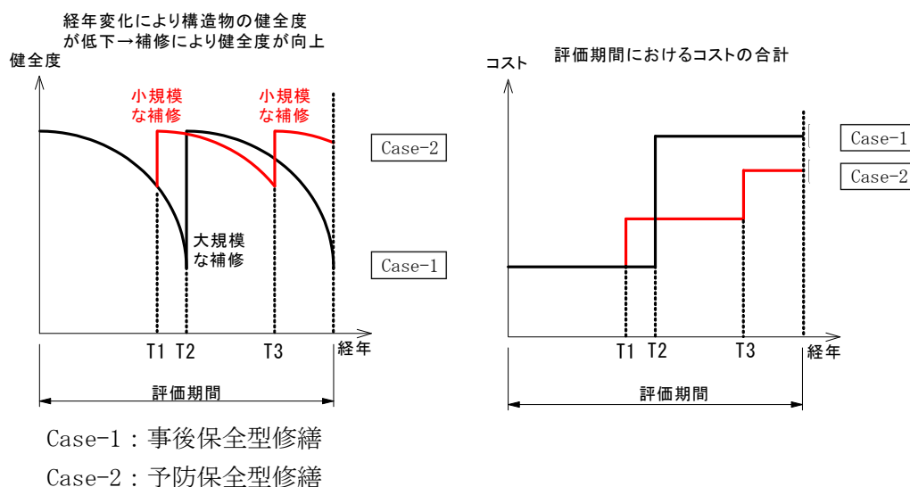
図-2.5.1 補修工事費設定のイメージ
