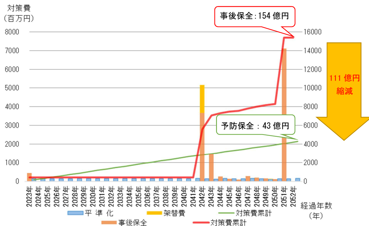
図-4.1.1 長寿命化修繕計画による縮減効果
