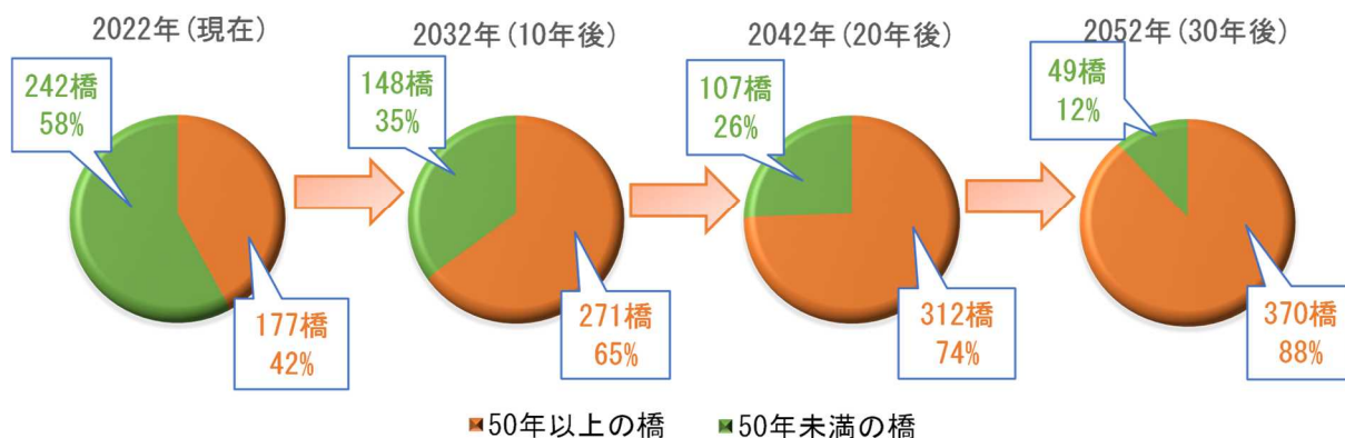
図-1.2.2 架設後 50 年以上施設の推移
